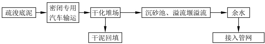
4-2 余水处理流程示意图
